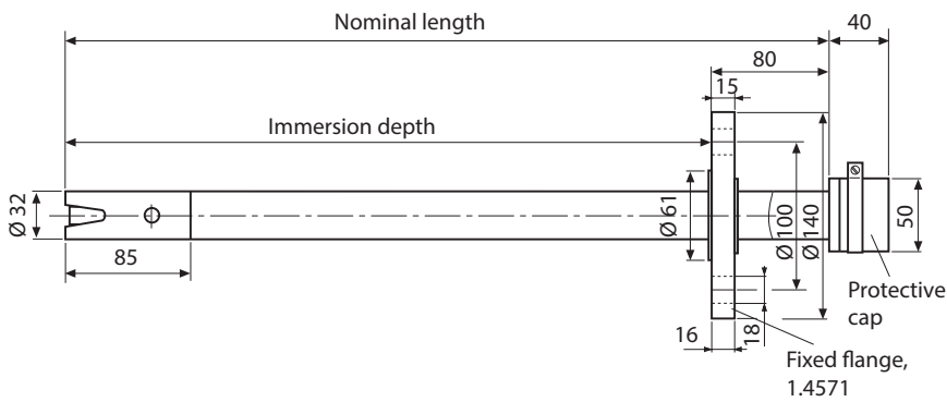
Flange, DN 32 PN 10/16
