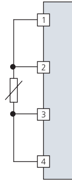
RTD 4 线电路
