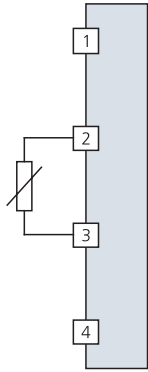
RTD 2 线电路
