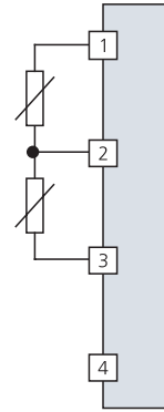
RTD 差分测量
