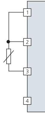
RTD 3 线电路
