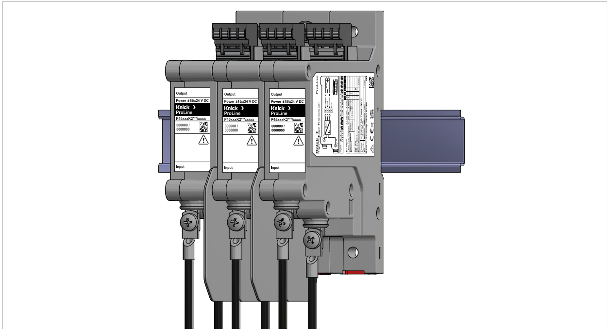
1 Push-in-Klemme 2 Schraubklemme
